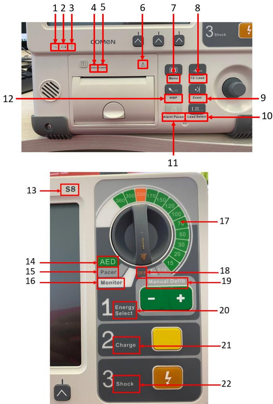
Рисунок 1.2.1.6 – Информация, нанесенная на переднюю сторону дефибриллятор-мониторов S6 и S8
